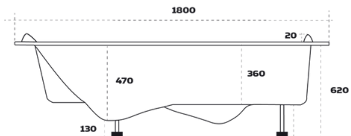
VUE EN COUPE (Dimensions exprimées en mm)
