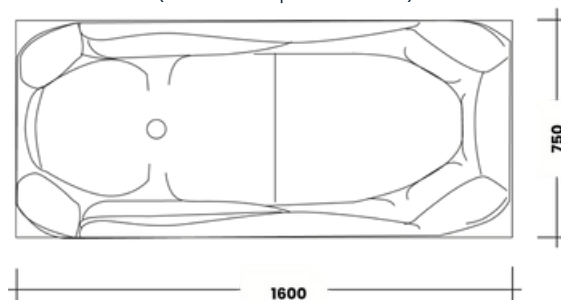
VUE DE DESSUS (Dimensions exprimées en mm)
