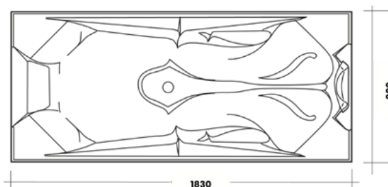
VUE DE DESSUS (Dimensions exprimées en mm)
