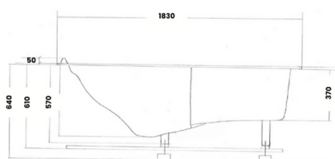
VUE EN COUPE (Dimensions exprimées en mm)
