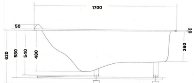
VUE EN COUPE (Dimensions exprimées en mm)
